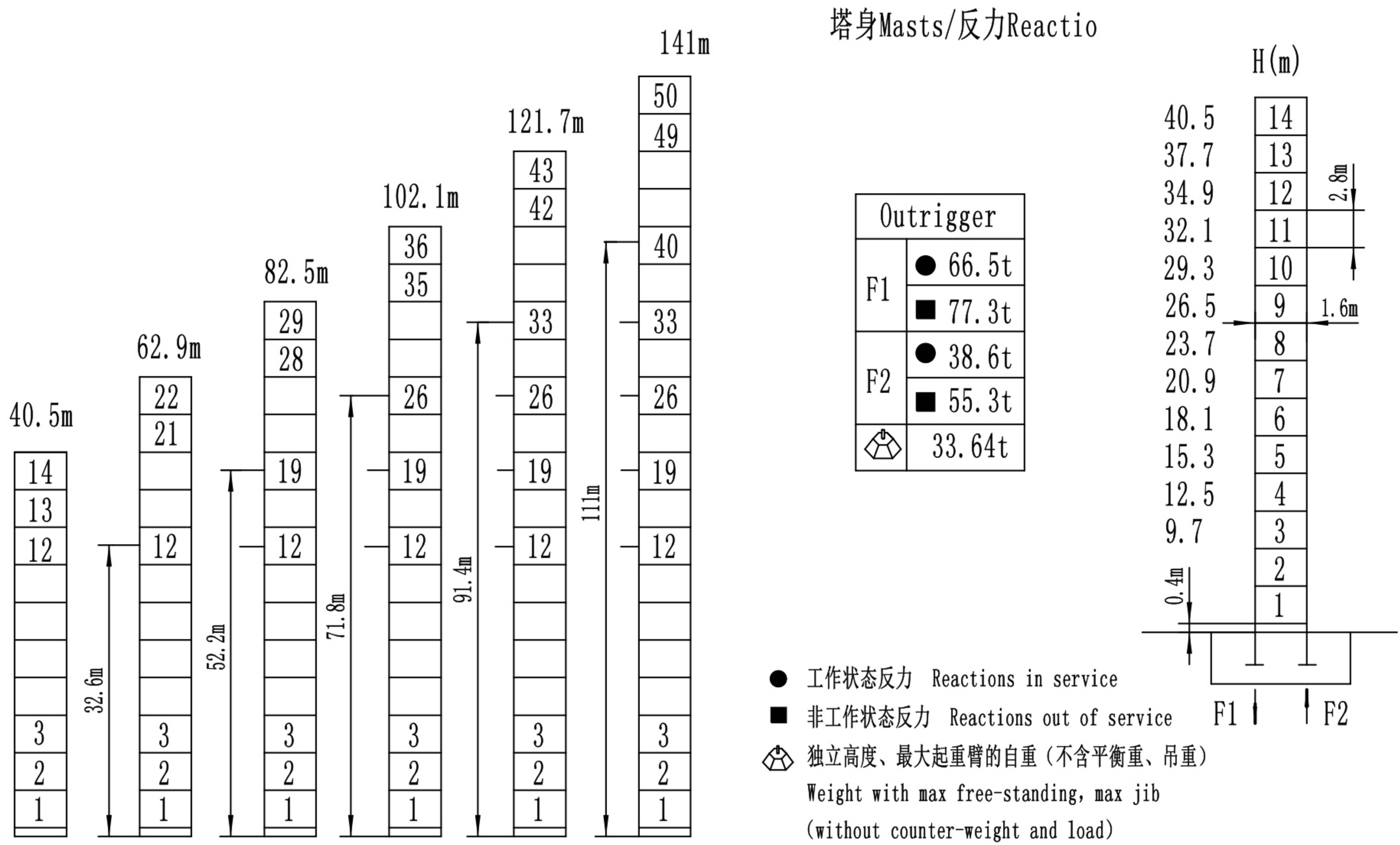
附着Anchorage
